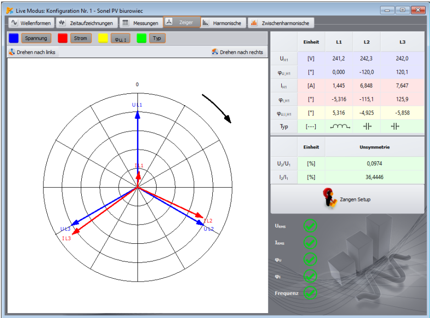
Abb. 50. Zeigerdiagramm für Sternschaltung.
