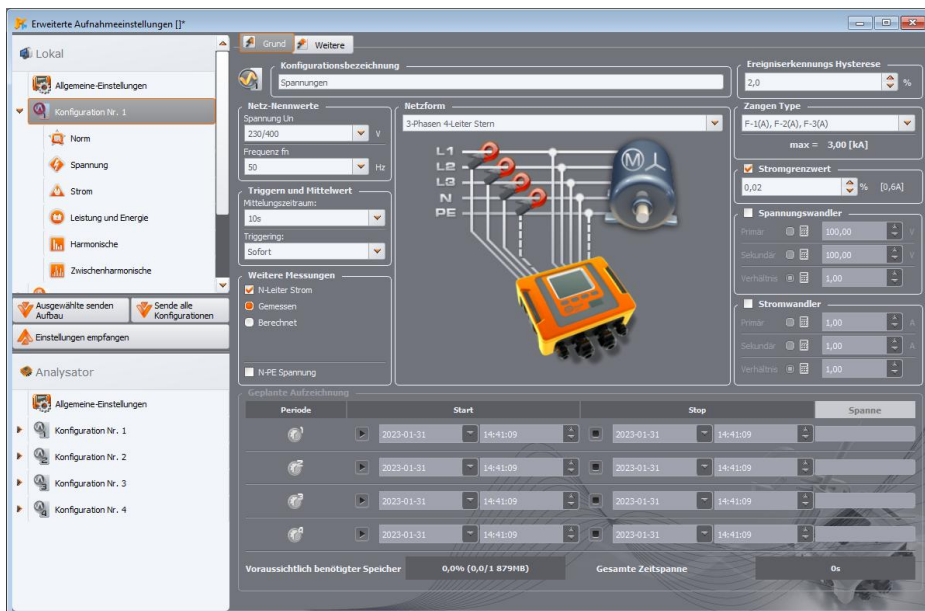
Abb. 16. Messkonfiguration – Hauptbildschirm und Einstellungsbaum.
