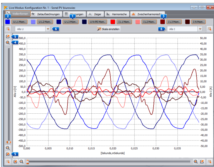
Abb. 46. Bildschirm im aktuellen Datenlesemodus - Wellenformen.
